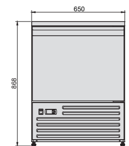
正视图 Front View
