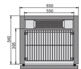
顶视图 Top view
