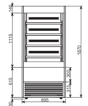
正视图 Front View
