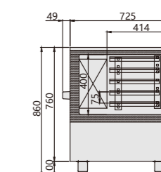
BC-5T(-32℃)
