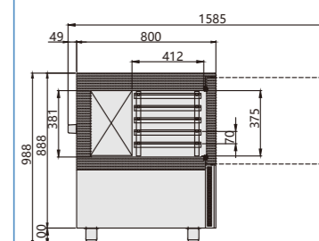
BC-5T(-40℃)
